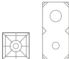
Feux vifs avec grille en fonte
